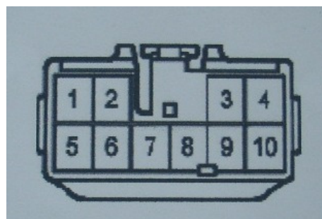
Connettore F45/F113
