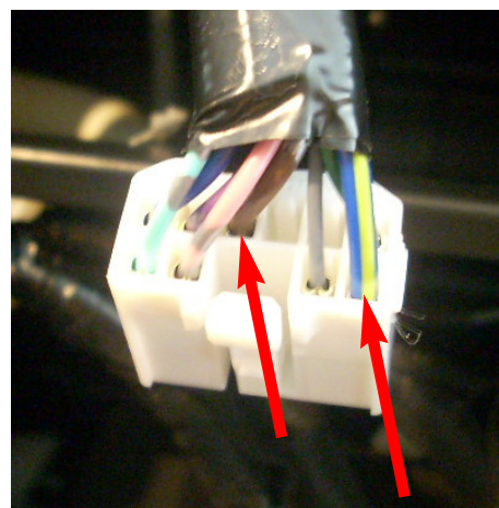
Connettore F45/F113
