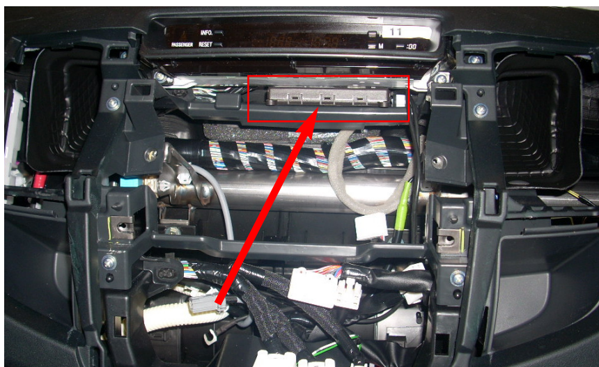
Connettore F45/F113
